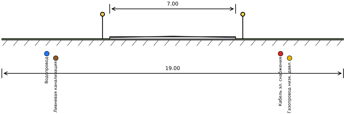
Разрез 1-1 (главный проезд)
