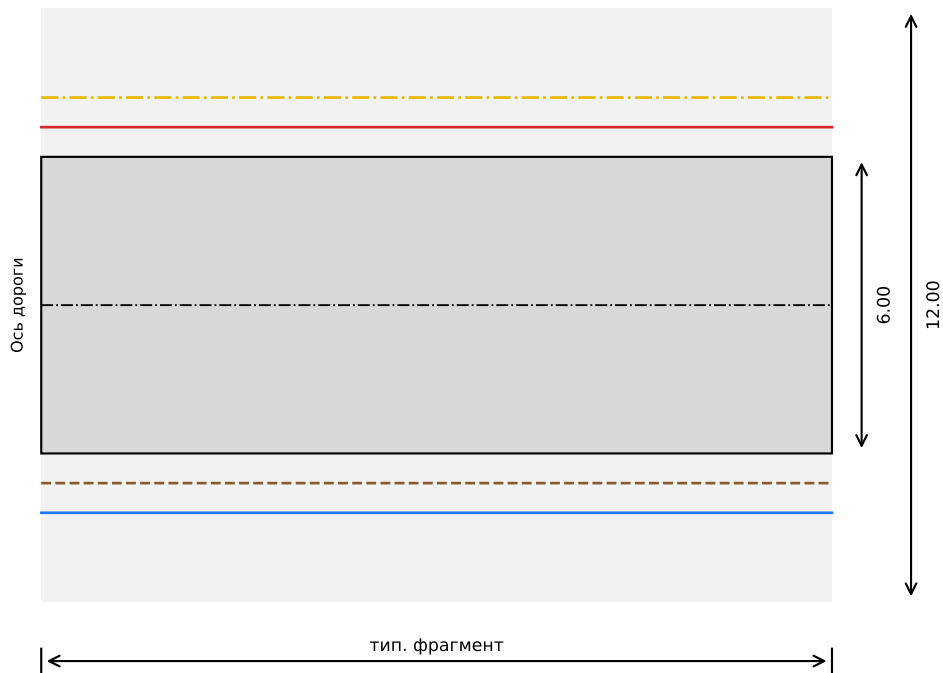
План дороги 2 (второстепенный)
