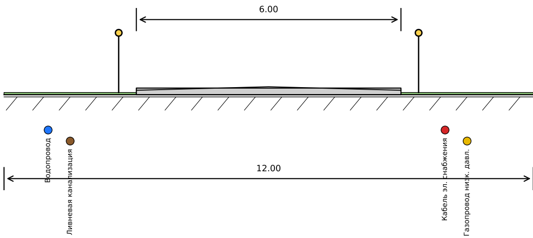
Разрез 2-2 (второстепенный)
